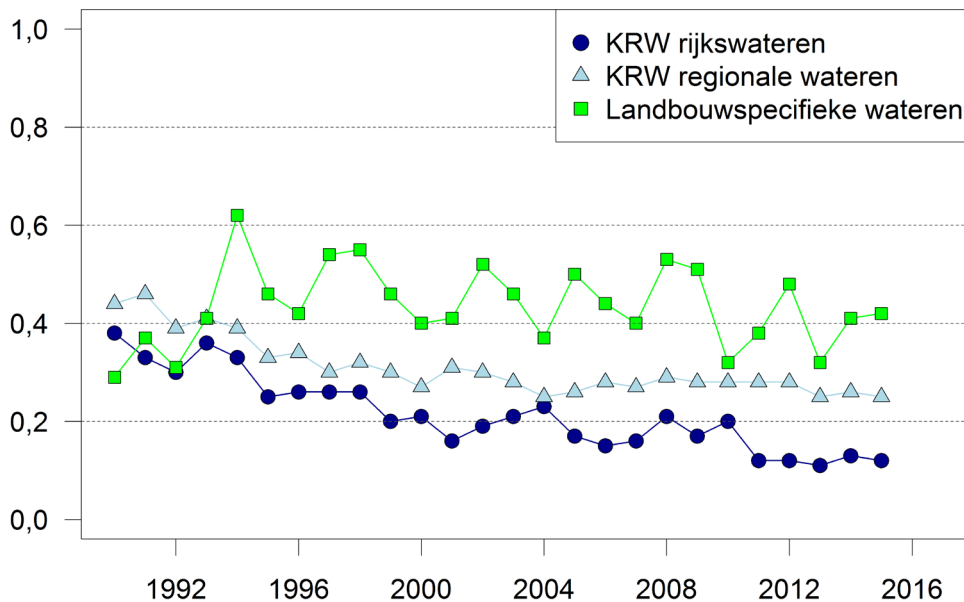
Figuur 3.6 Totaal-fosforconcentratie (zomergemiddelde als P in mg/l) in zoete wateren in de periode 1990-2015
