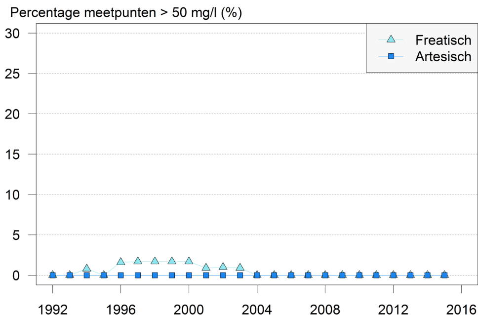
Figuur 2.14 Overschrijding van de EU-norm van 50 mg/l voor de gemiddelde nitraatconcentratie in het grondwater op drinkwaterproductielocaties voor freatisch grondwater en artesisch grondwater.
