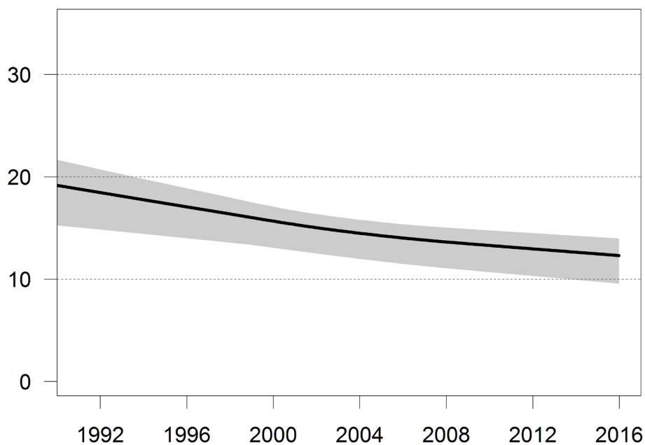
Figuur 3.9 Berekende trend in de nitraatconcentratie (wintermetingen; als \text{NO}_3 in mg/l) voor de KRW rijkswateren; mediane trend (doorgetrokken lijn) en het gebied tussen de 25- en 75-percentiel (grijs vlak)
