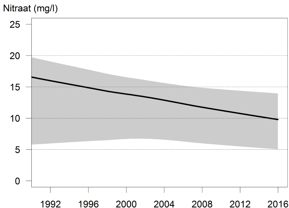
Figuur 4.5 Berekende trend voor de nitraatconcentratie (wintermetingen; als \text{NO}_3 in mg/l ) voor de KRW-overgangswateren; mediane trend (doorgetrokken lijn) en het gebied tussen de 25- en 75-percentiel trends (grijs vlak)
