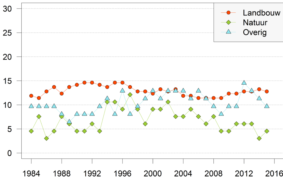
Figuur 2.3 Overschrijding van de EU-norm van 50 mg/l voor nitraat in het grondwater op een diepte van 5-15 m onder maaiveld per vorm van landgebruik
