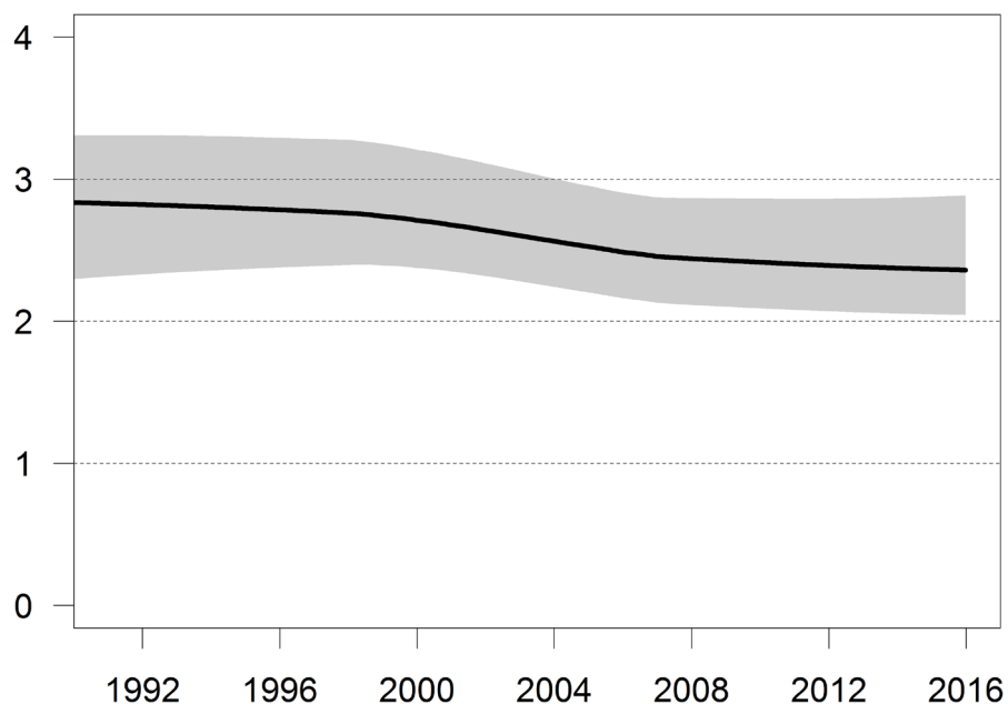
Figuur 4.6 Berekende trend voor nitraatconcentratie (wintermetingen; als NO 3 in mg/l) voor de kustwateren; mediane trend (doorgetrokken lijn) en het gebied tussen de 25- en 75-percentiel trends (grijs vlak)
