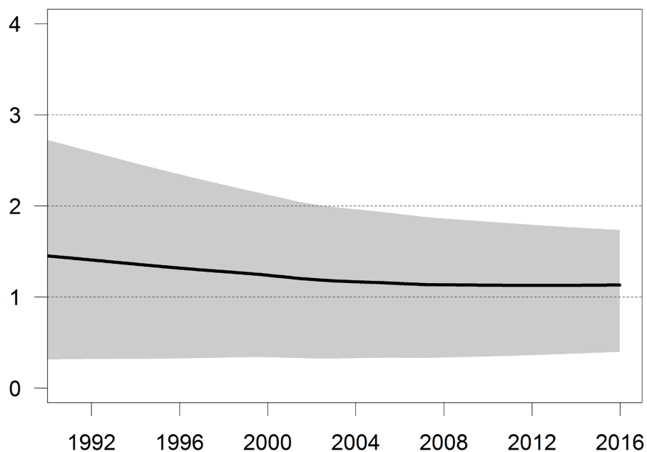
Figuur 4.7 Berekende trend voor nitraatconcentratie (wintermetingen; als NO 3 in mg/l) voor de open zee locaties; mediane trend (doorgetrokken lijn) en het gebied tussen de 25- en 75-percentiel (grijs vlak)
