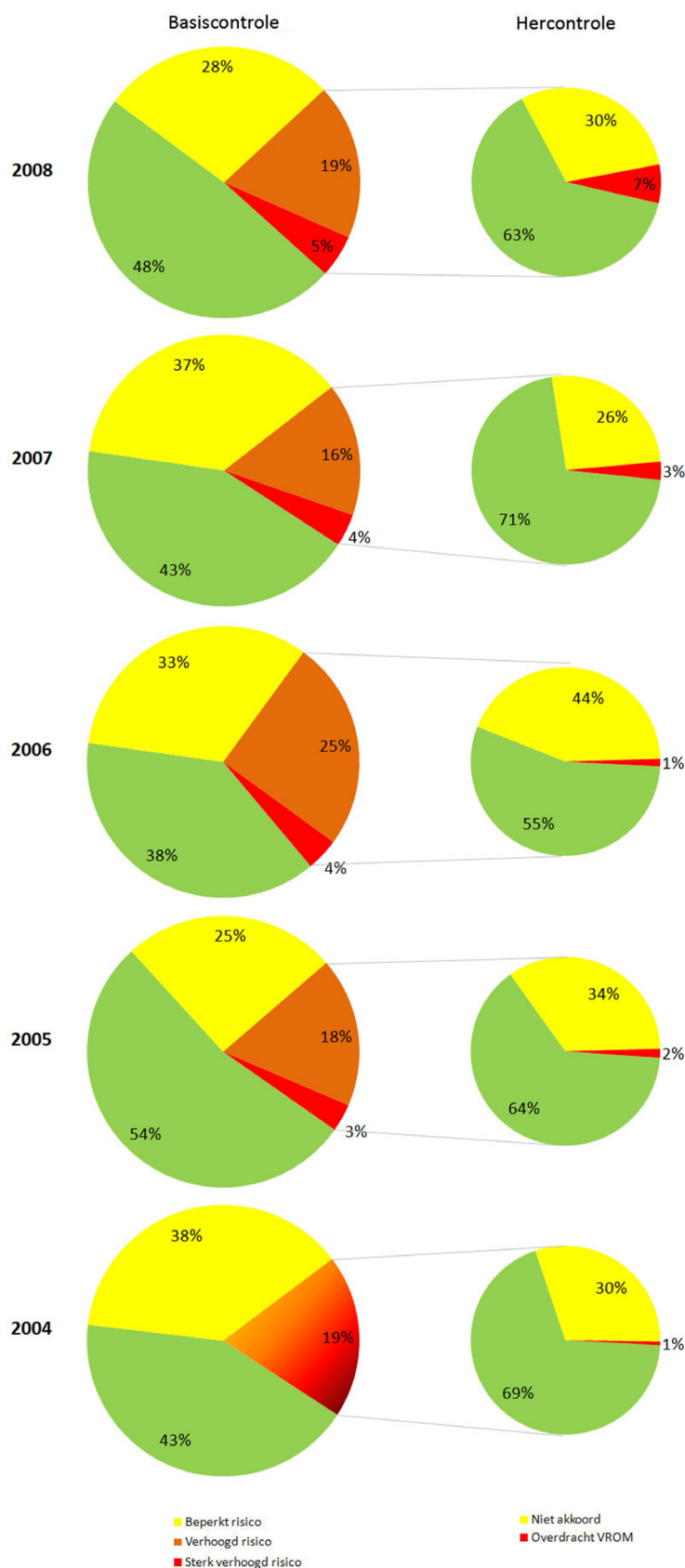
Figuur 2. Resultaten van de uitgevoerde controles in de bestaande bouw in de periode van 2004 - 2008. Het linkerdiagram presenteert de resultaten van de basiscontrole, het rechterdiagram presenteert de resultaten van de hercontrole bij installaties die bij basiscontrole gebreken met een (sterk) verhoogd risico vertonen. In 2004 is geen onderscheid gemaakt tussen verhoogd en sterk verhoogd risico (bron data 2004: rapportage Vewin).
