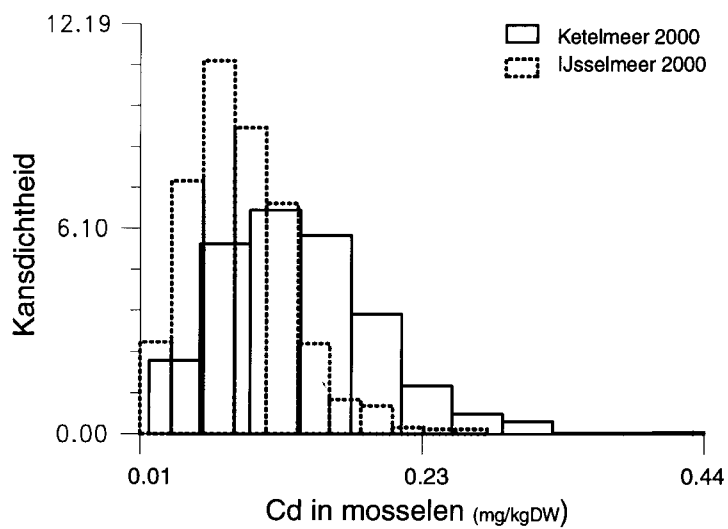
Figuur 17: Kansverdeling van cadmium in mosselen in Ketelmeer en IJsselmeer in het jaar 2000.
