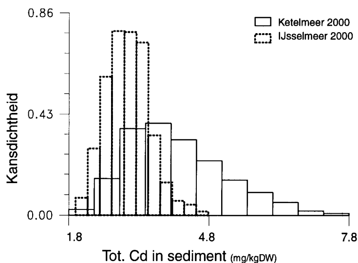
Figuur 15: Totaal Cd in nieuw gevormd sediment van Ketelmeer en IJsselmeer in het jaar 2000
