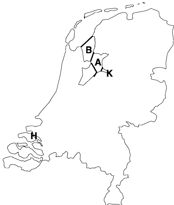
Fig 14: Ligging van de gemodelleerde gebieden. H = Hollands Diep/Haring Vliet (Traas et al. 1994), K = Ketelmeer, A = IJsselmeer, eerste segment, B = IJsselmeer, tweede segment.
