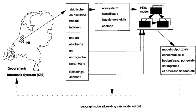
Fig. 5 Schema van parametrisering van CATS modellen voor specifieke ecosysteemtypen, c.q. gebieden.
