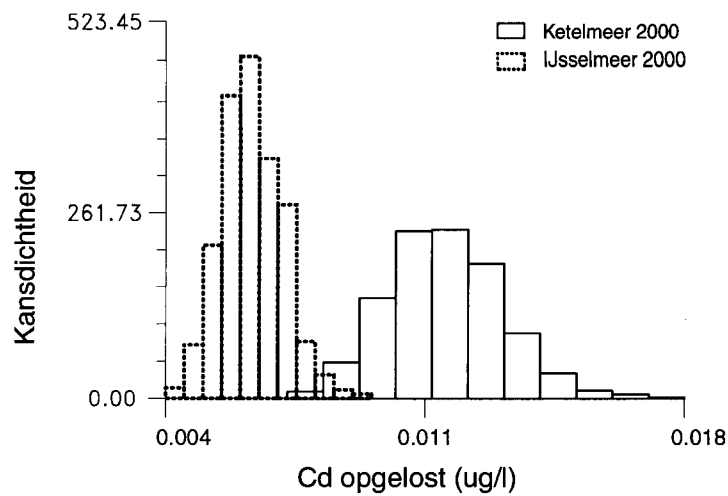
Figuur 16: Opgelost Cd in Ketelmeer en IJsselmeer (segment B) in het jaar 2000.
