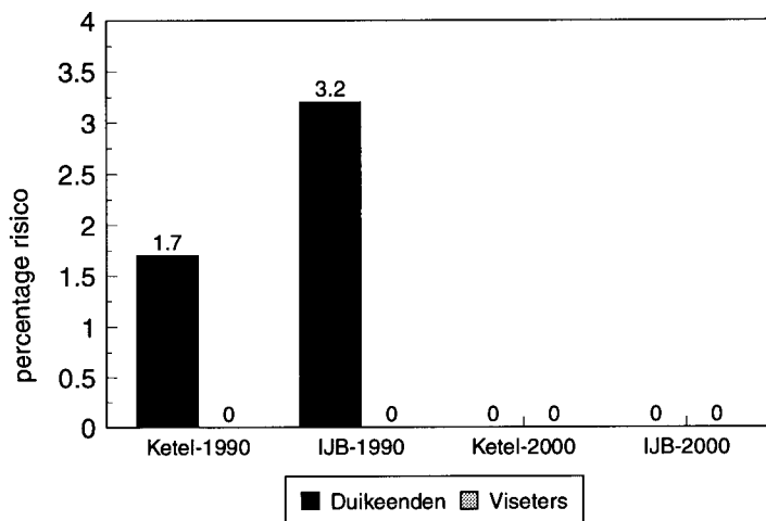
Figuur 22: Overschrijding van voedselkwaliteitsnormen voor eenden en viseters in het jaar 2000
