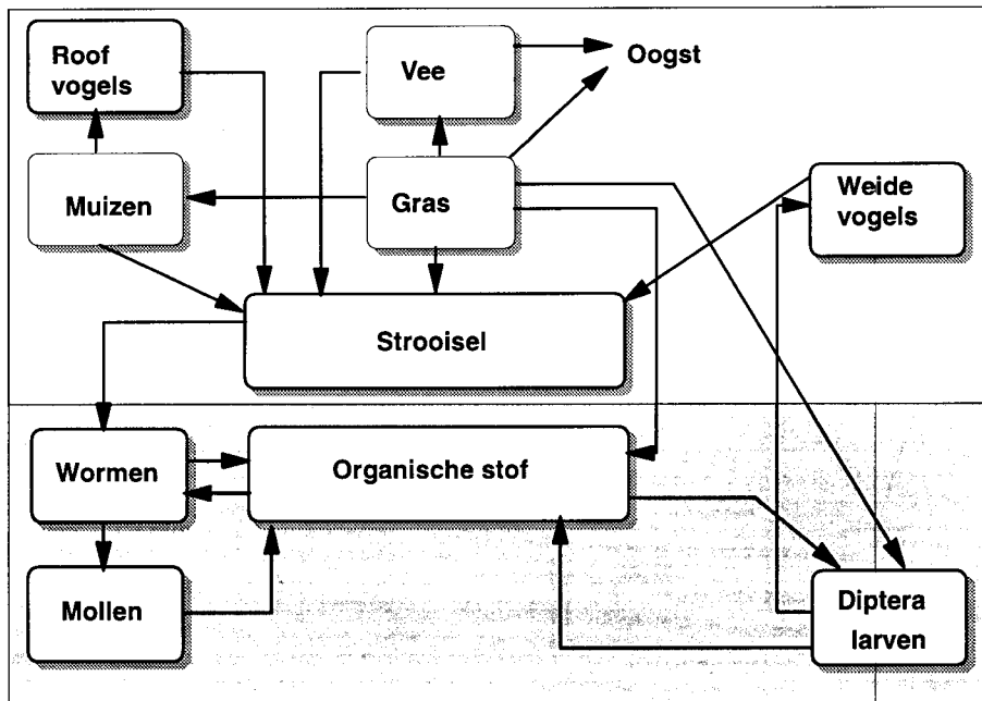
Figuur 1: Voedselwebstructuur van het CATS-1 model
