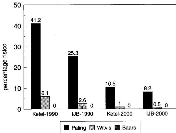
Figuur 21: Overschrijding van visconsumptienormen in het jaar 2000. IJB = IJsselmeer deel B.
