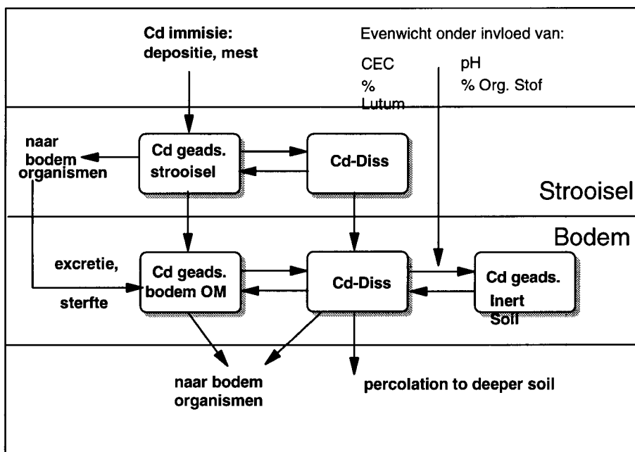
Figuur 2: cyclus van de toxische stof in CATS-1
