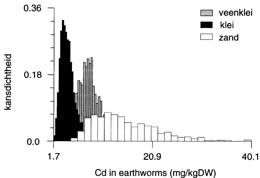
Figuur 11: Kansverdeling van de Cd conc. in regenwormen bij verschillende bodemtypes.
