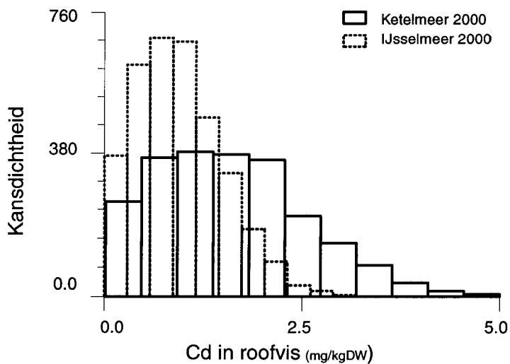
Figuur 18: Kansverdeling van cadmium in roofovis in Ketelmeer en IJsselmeer in het jaar 2000.
