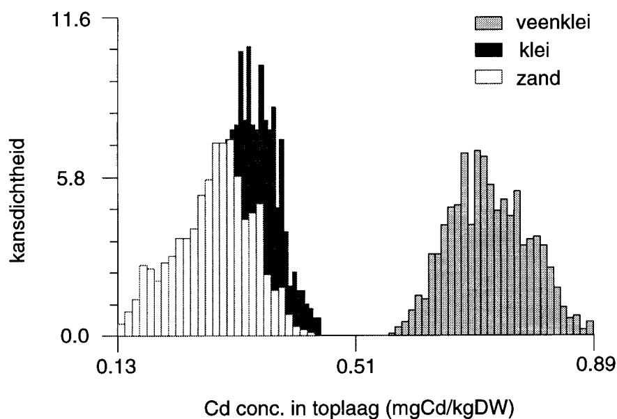
Figuur 9: Kansverdeling van de Cd conc. in de toplaag, bij verschillende bodemtypes.
