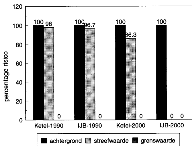
Figuur 19: Kans op overschrijding van normen voor Cd-opgelost in de jaren 1990 en 2000. IJB = IJsselmeer, deel B.
