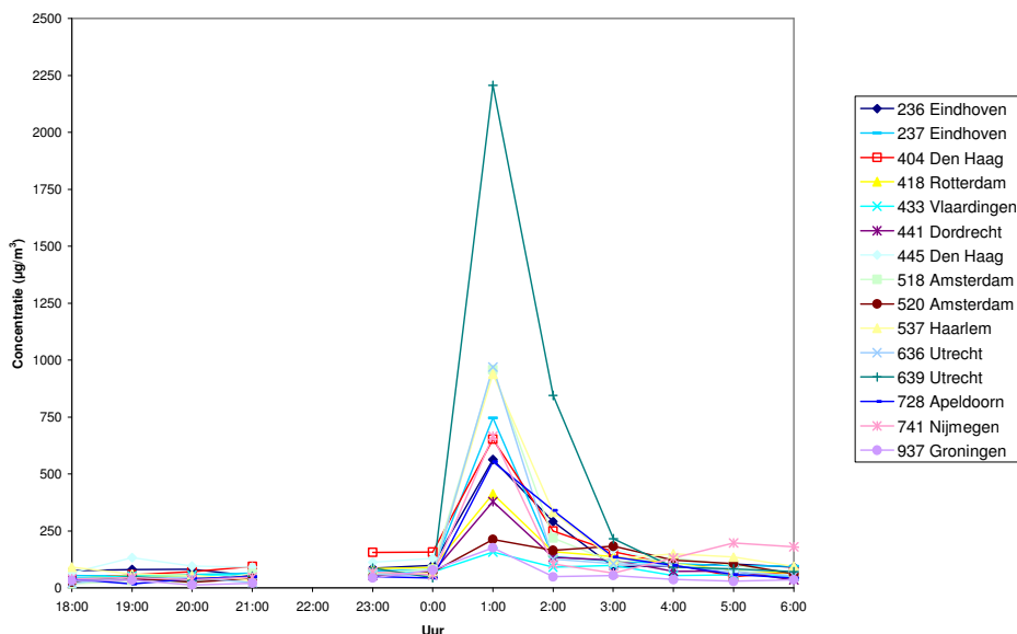
Figuur 1: Uurgemiddelde concentratie fijn stof in stedelijk gebied tijdens de jaarwisseling van 2003/2004.
