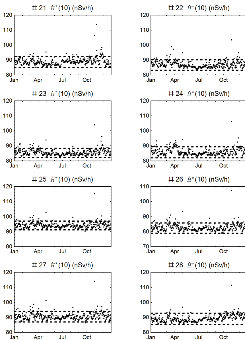
Figuur 4 Het daggemiddelde omgevingsdosis-equivalenttempo \dot{H}^*(10) voor de MONET-monitoren rond EPZ/KCB in 2018 uit Figuur 3 samen met, als gestippelde lijnen, de variatie van de natuurlijke achtergrond, bepaald met de methode beschreven in paragraaf 3.3. De figuur voor monitor 26 heeft een andere schaalverdeling voor de y-as.
