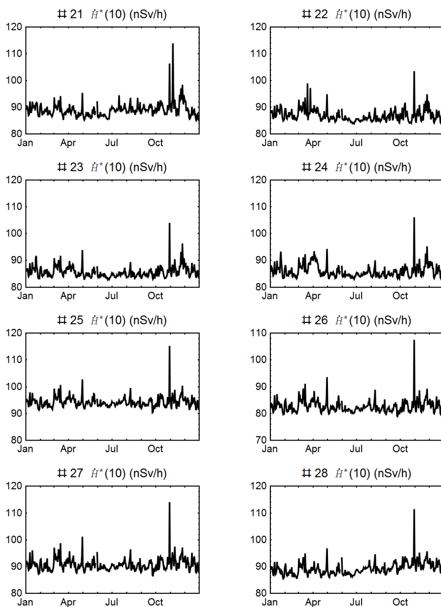
Figuur 3 Het gemeten daggemiddelde omgevingsdosisequivalenttempo voor de MONET-monitoren rond EPZ/KCB in 2018. De figuur voor monitor 26 heeft een andere schaalverdeling voor de y-as. Op 30 oktober 2018, de dag met maximum neerslag in 2018, registreren alle monitoren een verhoogde \dot{H}^*(10) .
