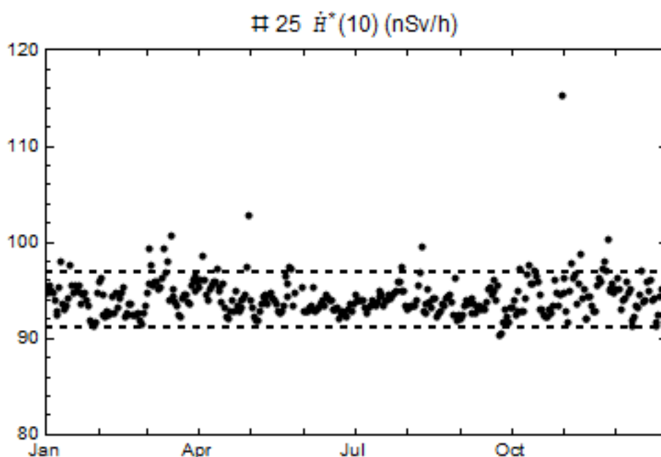
Figuur 5 Het gemeten omgevingsdosisequivalenttempo voor monitor 25 bij EPZ/KCB in 2018 (uit Figuur 4), samen met, als gestippelde lijnen, de natuurlijke achtergrond en de spreiding ervan over het jaar.
