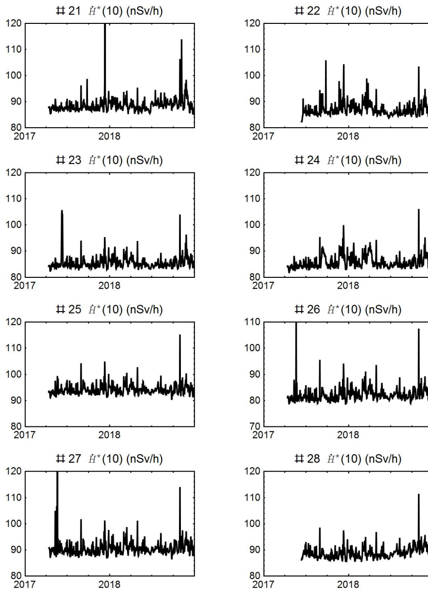
Figuur B1.1 Verloop van het omgevingsdosis-equivalenttempo (daggemiddelden) in 2017 en 2018. De figuur voor monitor 26 heeft een andere schaalverdeling voor de y-as.
