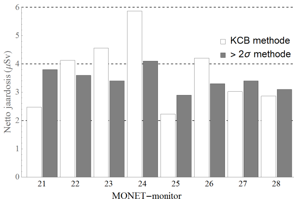
Figuur 7 Vergelijking tussen de jaardosis voor het jaar 2018 bepaald volgens de EPZ/KCB-mediaan- en de MONET ' >2\sigma '-methode toegepast op daggemiddelden.
