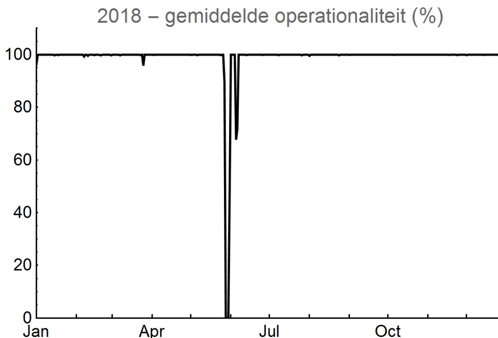
Figuur 2 Operationaliteit per dag van MONET rond EPZ/KCB in 2018, gemiddeld over de acht monitoren.
