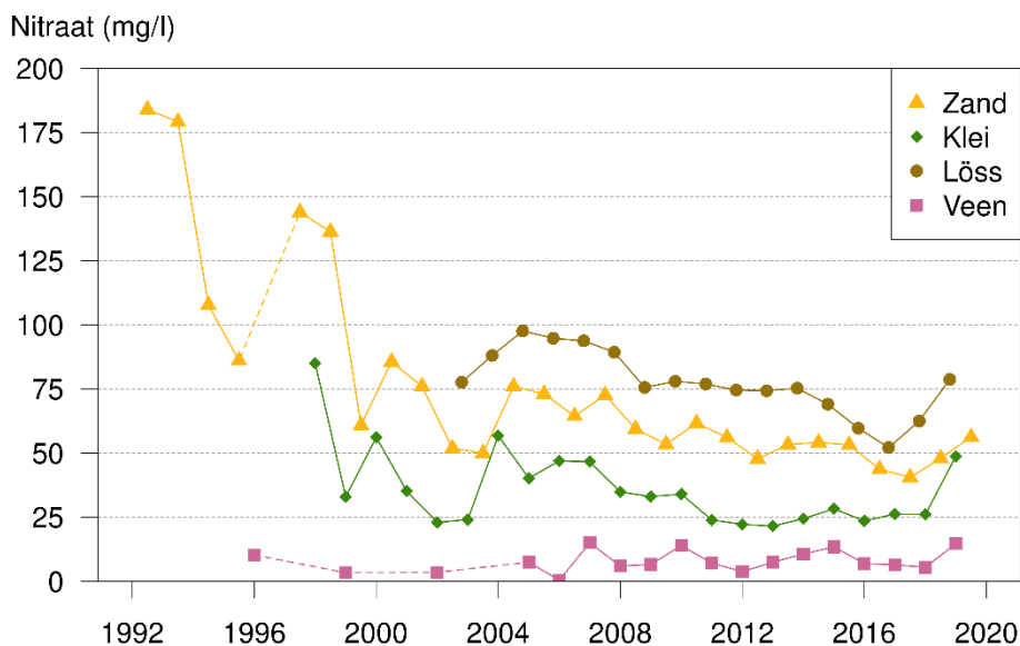
Figuur S2 Nitraatconcentratie (als NO 3 in mg/l) in het water dat uitspoelt uit percelen op landbouwbedrijven per regio in de periode 1992-2019. Weergegeven is de jaargemiddelde concentratie.
