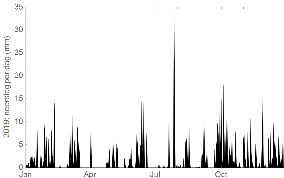
Figuur 6 Neerslag per dag, in mm, gemeten door het KNMI weerstation van Vlissingen (bron: KNMI). Hevige neerslag op 27 januari, 10 februari, 7 maart, 27 en 28 juli en 28 november valt samen met een verhoging van \dot{H}^*(10) van alle monitoren van het EPZ/KCB MONET-meetnet.
