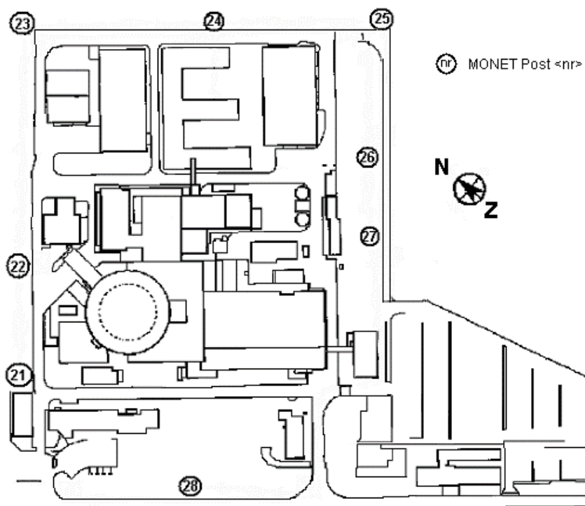
Figuur 1 Overzicht van de terreinopstelling van de kerncentrale te Borssele. De doorsnede van het reactorgebouw is 40 m. De centrale post van het MONET meetnet staat vanaf 2017 in gebouw 74.
