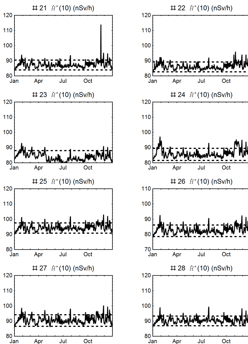
Figuur 4 Het daggemiddelde omgevingsdosis-equivalenttempo \dot{H}^*(10) voor de MONET-monitoren rond EPZ/KCB in 2019 uit Figuur 3 samen met, als gestippelde lijnen, de variatie van de natuurlijke achtergrond, bepaald met de methode beschreven in paragraaf 3.3. De figuur voor monitor 26 heeft een andere schaalverdeling voor de y-as.
