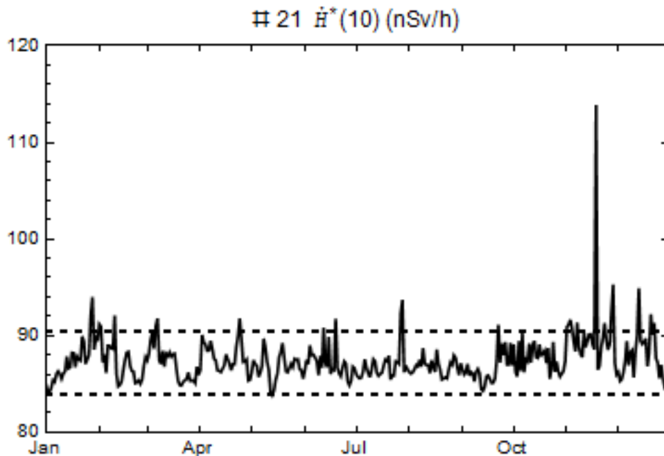
Figuur 5 Het gemeten omgevingsdosis-equivalenttempo voor monitor 21 bij EPZ/KCB in 2019 (uit Figuur 4), samen met, als gestippelde lijnen, de natuurlijke achtergrond en de spreiding ervan over het jaar.
