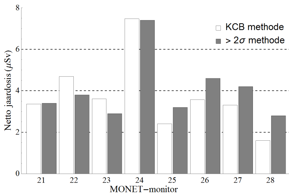
Figuur 7 Vergelijking tussen de jaardosis voor het jaar 2019 bepaald volgens de EPZ/KCB-mediaan- en de MONET '>2σ'-methodetoegepast op daggemiddelden.
