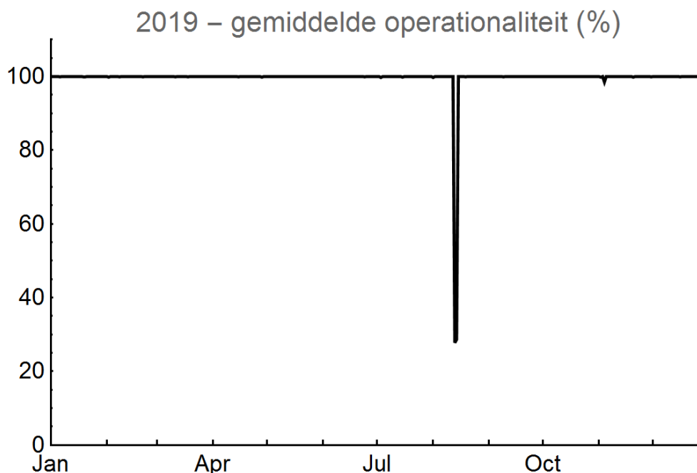
Figuur 2 Operationaliteit per dag van MONET rond EPZ/KCB in 2019, gemiddeld over de acht monitoren.
