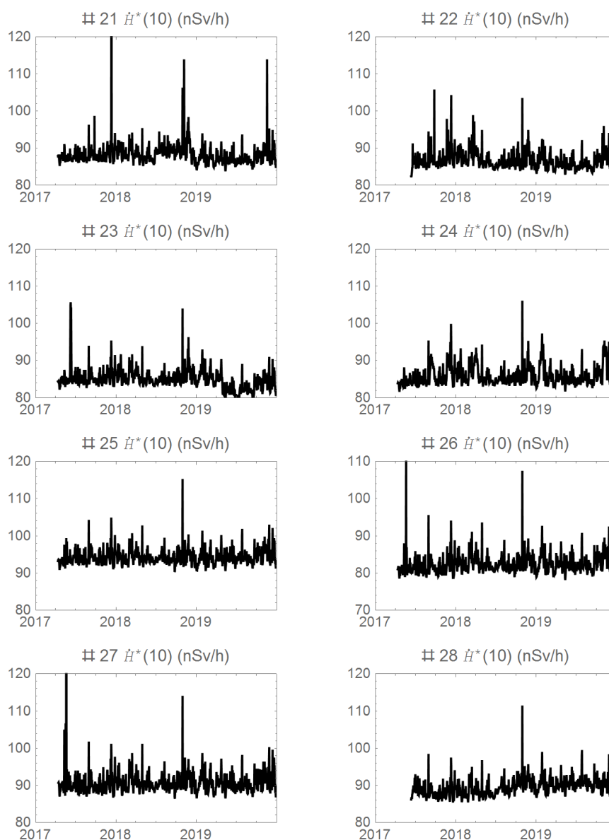
Figuur B1.1 Verloop van het omgevingsdosis-equivalenttempo (daggemiddelden) tussen 2017 en 2019. De figuur voor monitor 26 heeft een andere schaalverdeling voor de y-as.
