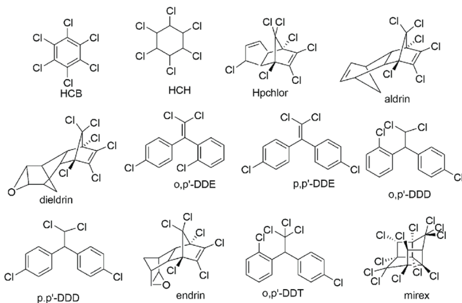
Figuur 8 Moleculaire structuur van enkele organochloor werkzame stoffen.
