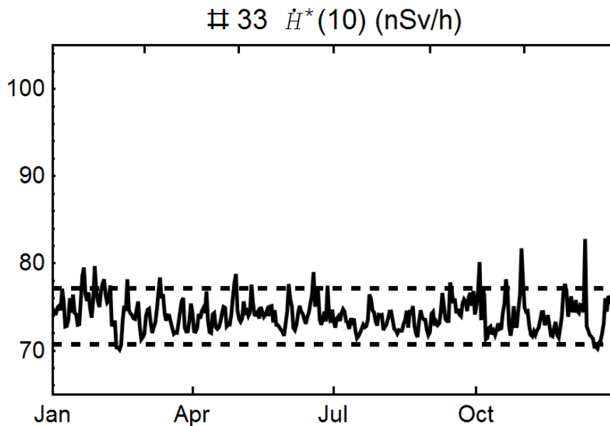
Figuur 5 Het gemeten omgevingsdosis-equivalenttempo voor monitor 33 in 2021 (uit Figuur 3) samen met de natuurlijke achtergrond en de spreiding als gestippelde lijnen over het jaar. De pieken op 10 december en op 3, 30 en 31 oktober 2021 vallen samen met hevige neerslag.
