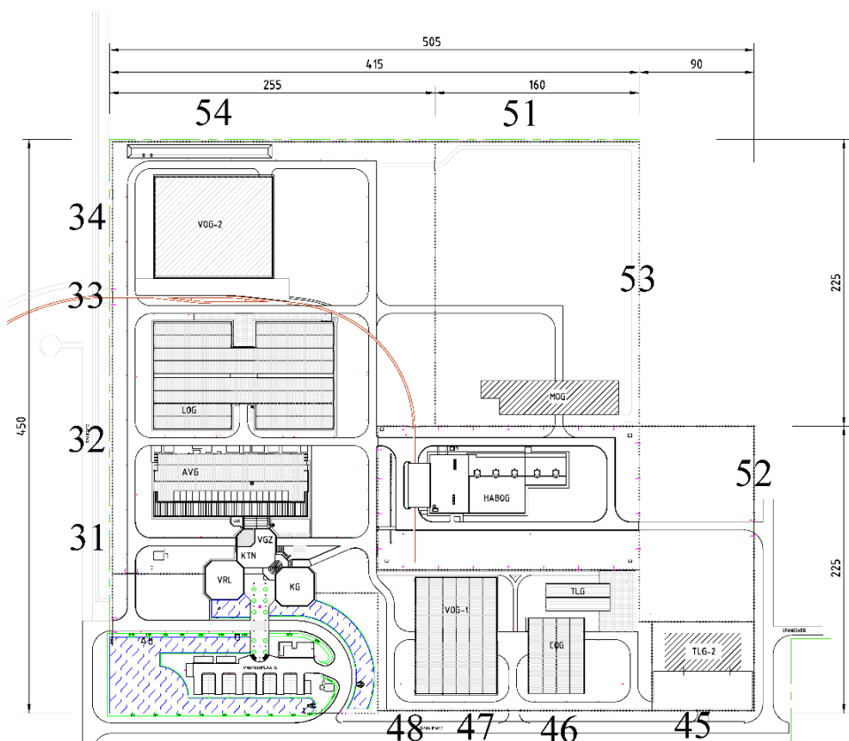
Figuur 1 Overzicht terreinopstelling COVRA met de locaties van de MONET meetposten vanaf 10 april 2015.
