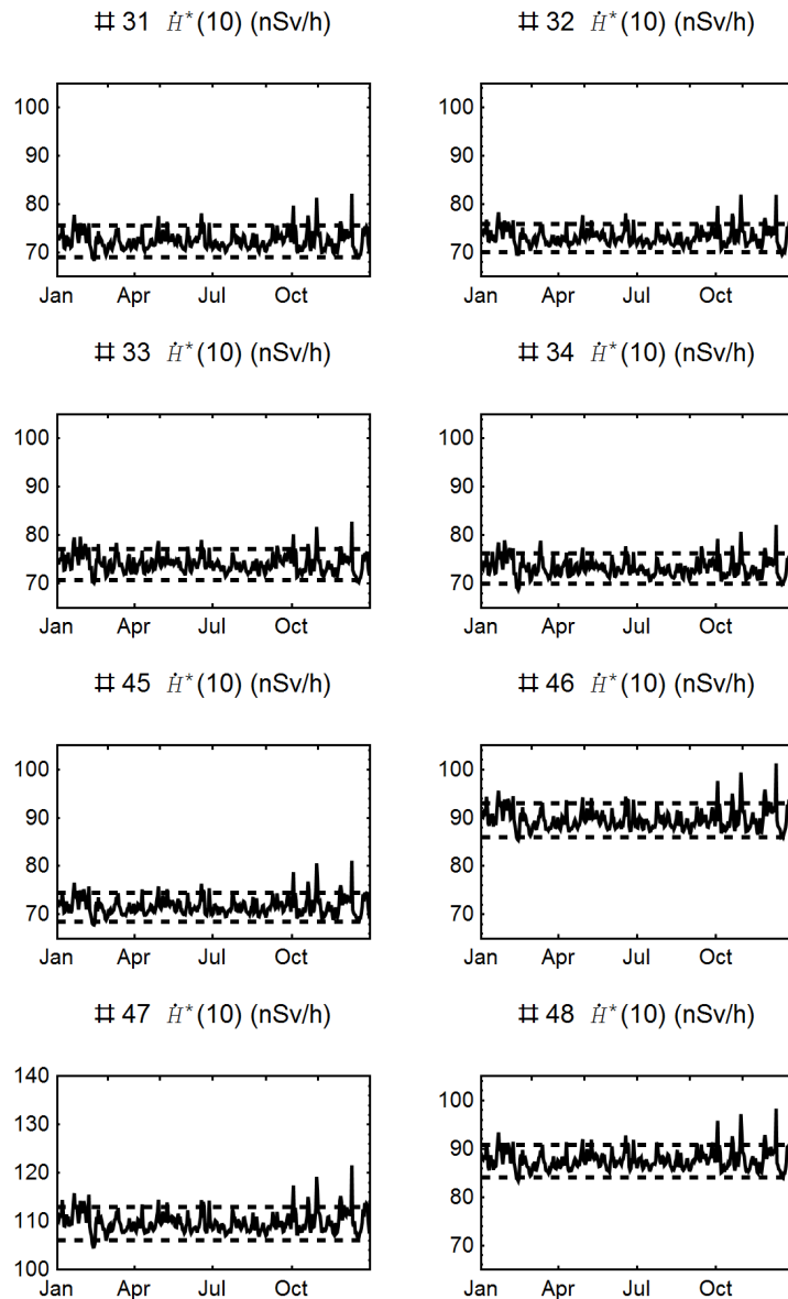
Figuur 3 Het daggemiddelde omgevingsdosis-equivalenttempo \dot{H}^*(10) voor de MONET-monitoren M31-M34 en M45-M48 aan de terreingrens van COVRA in 2021 samen met, als gestippelde lijnen, de variatie van de natuurlijke achtergrond. De figuur voor monitor 47 heeft een andere schaalverdeling voor de y as.
