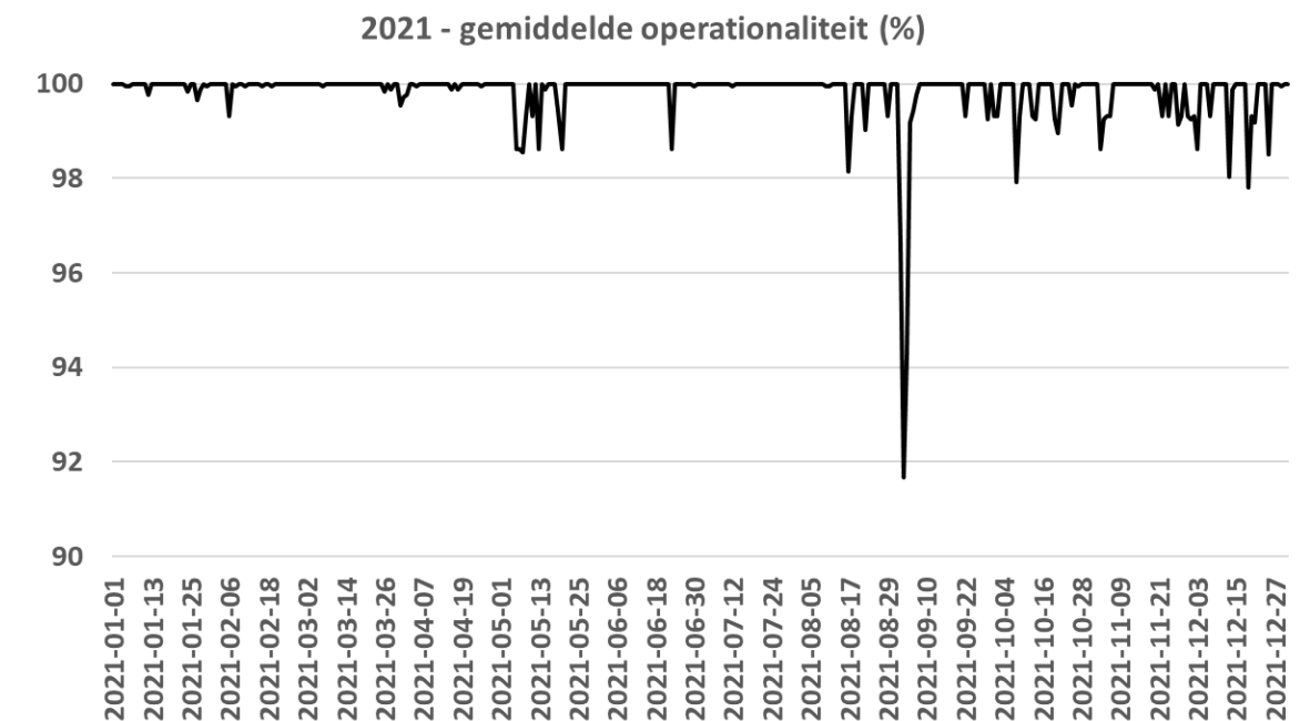
Figuur 2 Gemiddelde operationaliteit per dag van MONET aan de terreingrens van COVRA in 2021.
