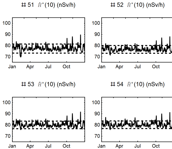
Figuur 4 Het daggemiddelde omgevingsdosis-equivalenttempo \dot{H}^*(10) voor de MONET-monitoren M51-M54 aan de terreingrens van COVRA in 2021 samen met, als gestippelde lijnen, de variatie van de natuurlijke achtergrond.
