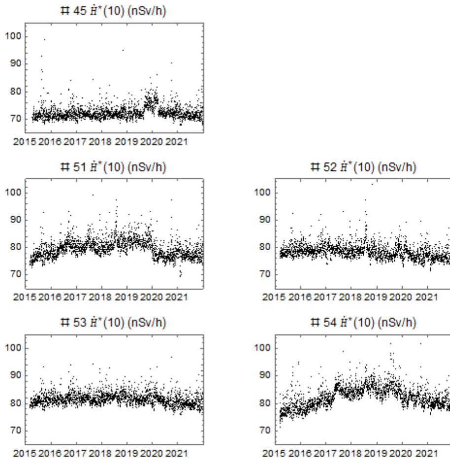
Figuur 8 Verloop van het daggemiddelde omgevingsdosistempo vanaf het jaar 2015 voor de nieuw geplaatste meetposten 51 t/m 54, en van meetpost 45, die in 2015 verplaatst is.
