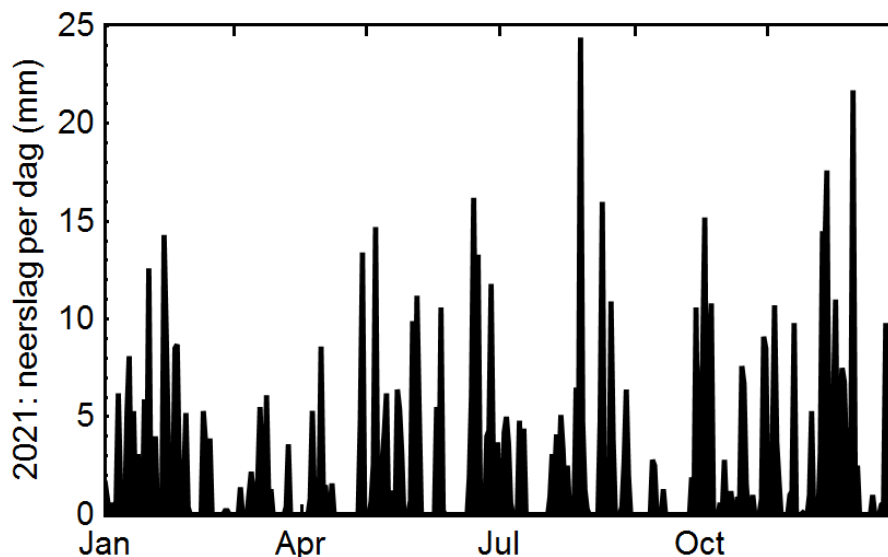
Figuur 6 Neerslag per dag, in mm, gemeten door het KNMI weerstation van Vlissingen (bron: KNMI). Hevige neerslag op 10 december en op 3, 30 en 31 oktober 2021 valt samen met een verhoging van het omgevingsdosis-equivalenttempo van alle monitoren van het MONET-meetnet.
