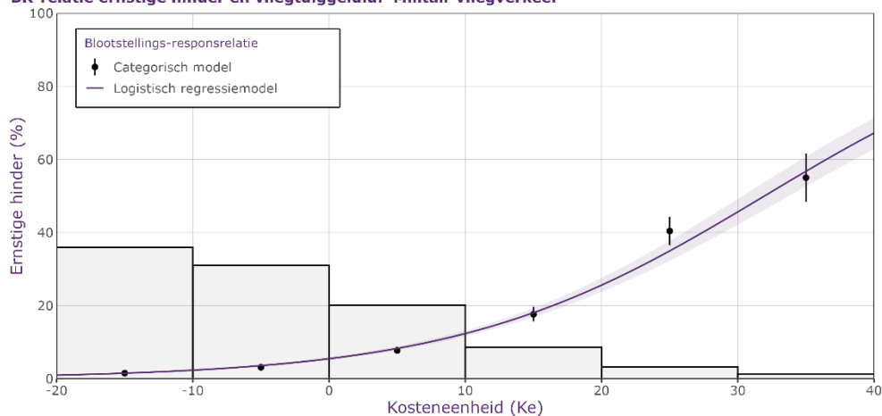
Figuur B2.1 Blootstelling-responsrelatie (BR-relatie) tussen ernstige hinder en blootstelling aan vliegtuigeluid (Kosteneenheid, berekend met NRM binnen de studiegebieden van militaire luchthavens.
