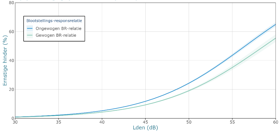
Figuur 5.3 Vergelijking ongewogen en gewogen Blootstelling-responsrelatie (BR-relatie) tussen ernstige hinder en blootstelling aan vliegtuigeluid ( L_{den} , berekend met Doc29 of Nederlands Rekenmodel (NRM)) rondom Schiphol Airport, Rotterdam The Hague Airport en Vliegbasis Volkel.
