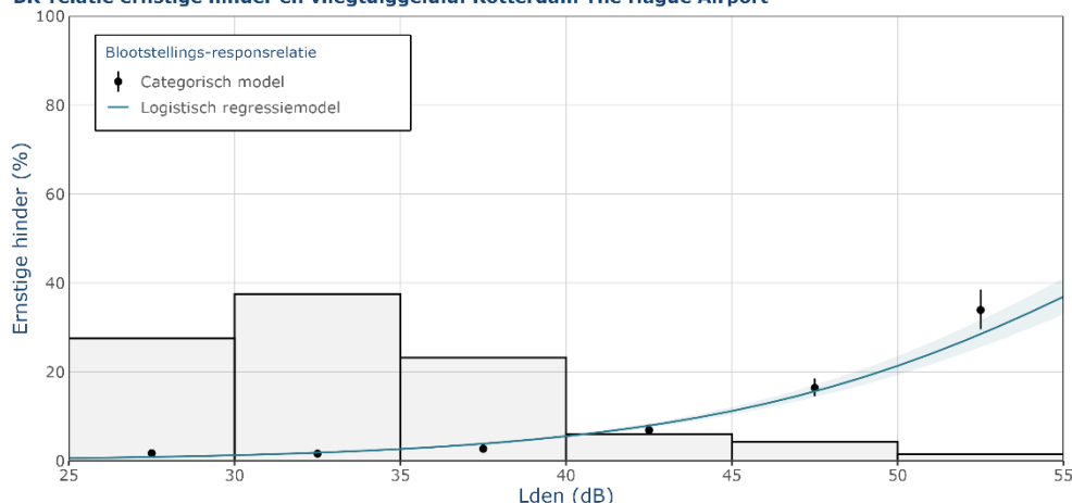
BR-relatie ernstige hinder en vliegtuigeluid: Rotterdam The Hague Airport
