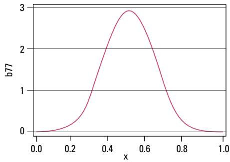
Bèta(7,7); prior voor alle Se
