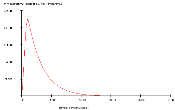
Figuur 8: blootstelling toilet 2,5 m 3 , ventilatievoud 1,5 h -1
