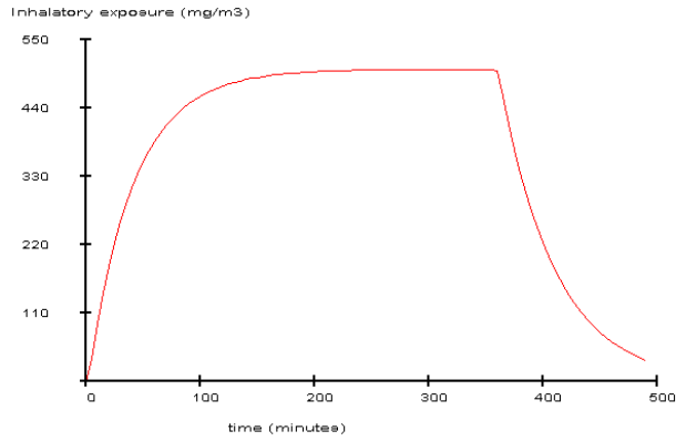
Figuur 5: blootstelling woonkamer 58 m 3 , ventilatievoud 1,5 h -1
