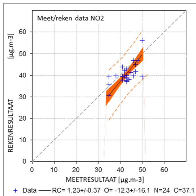
Figuur B6.2 Berekende en gemeten NO 2 -concentraties in straattype 2.
