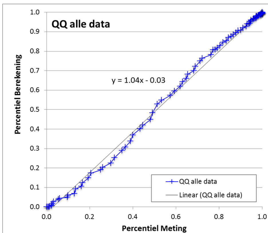
Figuur B5.2 Quantile/Quantile-plot van de gemeten en berekende NO 2 -concentraties.
