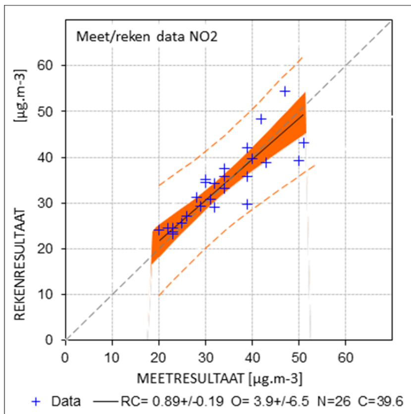
Figuur B4.8 Gemeten en berekende \text{NO}_2 -concentraties in 2011 op de meetlocaties van de gemeente Nijmegen.
