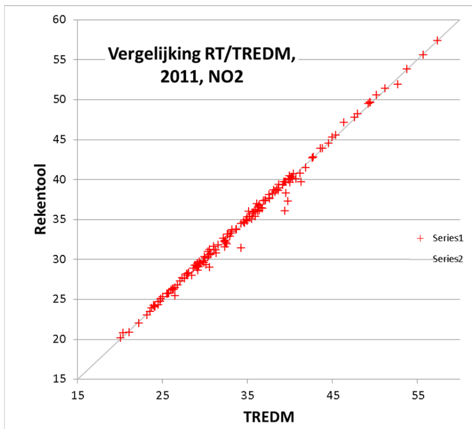
Figuur 3.1 Vergelijking tussen met de NSL-Rekentool en met TREDM berekende NO 2 -concentraties.
