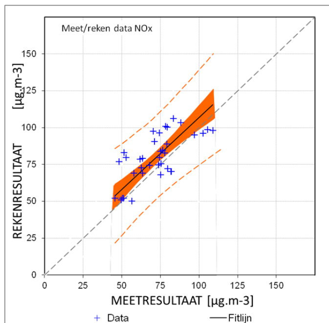
Figuur 5.8 Plot van gemeten en met gekalibreerde modelparameters berekende NO x -concentraties op straatstations in het LML (2009-2011) en DCMR-meetnet (2010-2011).
