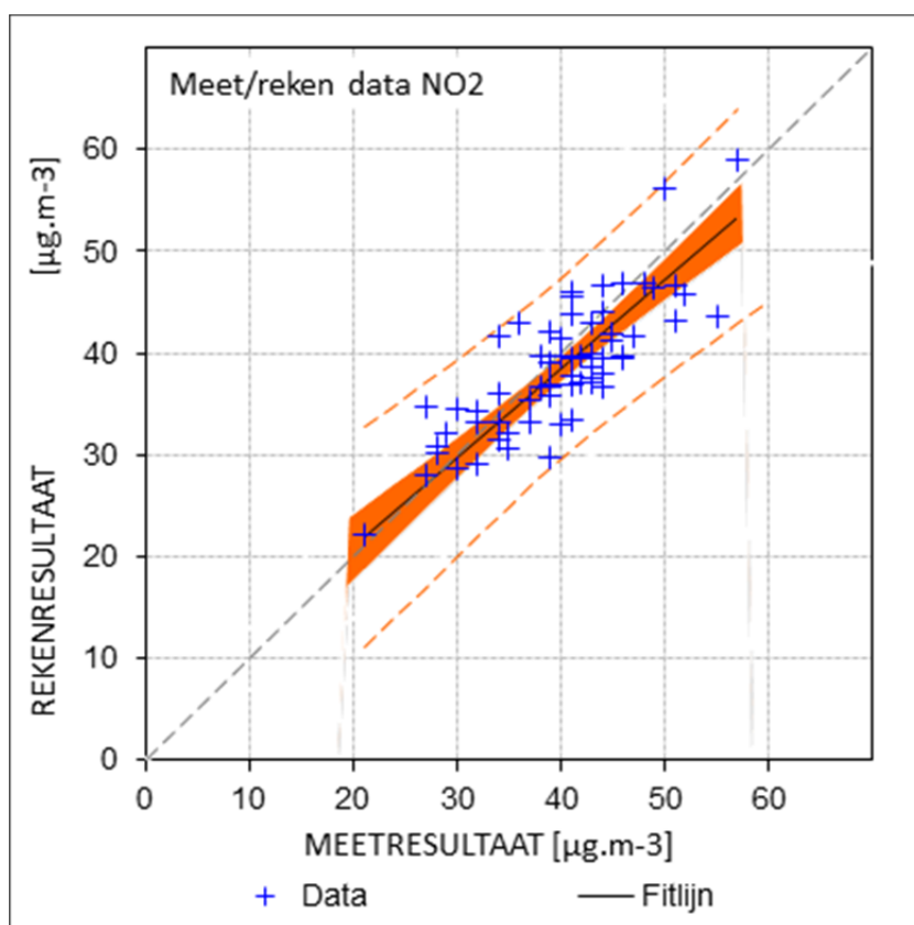
Figuur 4.9 Gemeten en berekende NO 2 -concentraties op stedelijke locaties in straten zonder gemodelleerde invloed van bomen.
