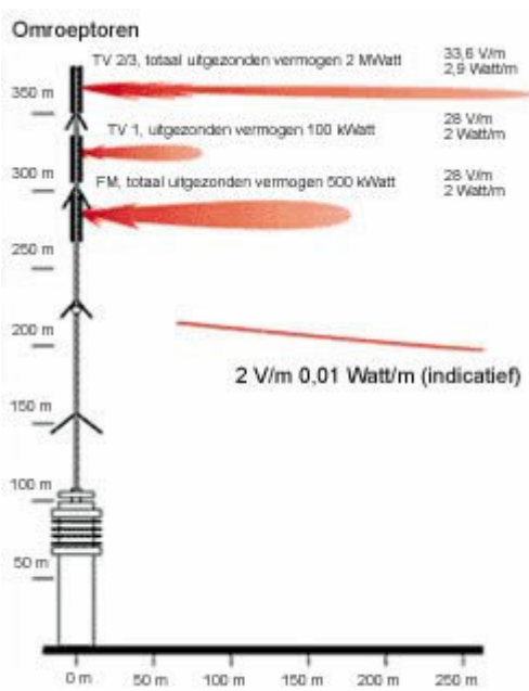
Voorbeeld van omroepstoren met zenders voor FM en TV. In de figuur is aangegeven binnen welke afstand van de antennes de limietwaarden van de Gezondheidsraad overschreden worden. (Bron: Antennebureau, 2002)
