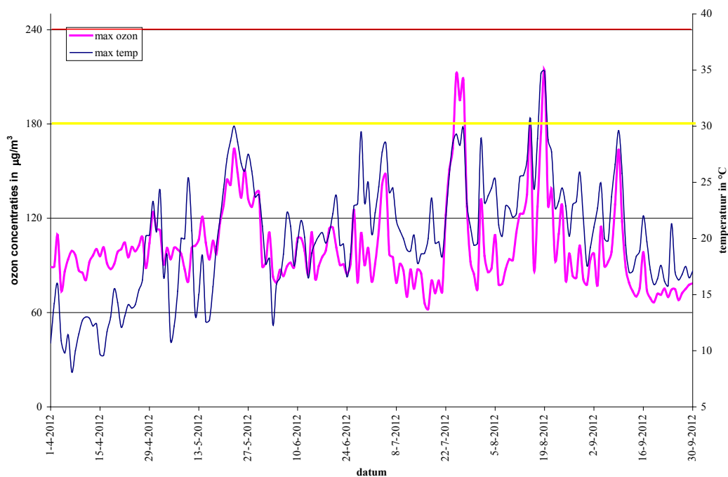
Figuur 1: Landelijke maximum ozonconcentratie en maximum temperatuur in de zomer van 2012
